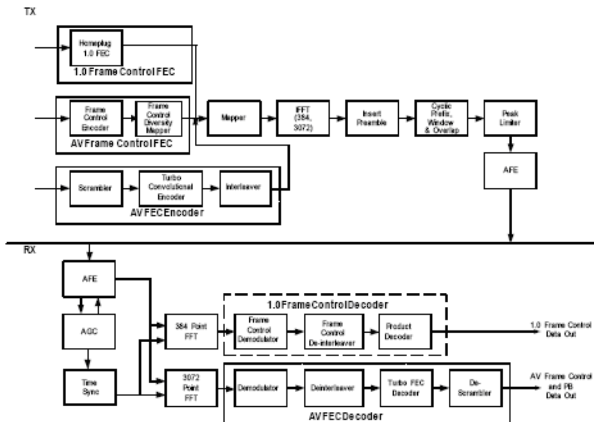
Рис.2.4 Структурна схема приймача-передавача для реалізації HomePlug v.AV
