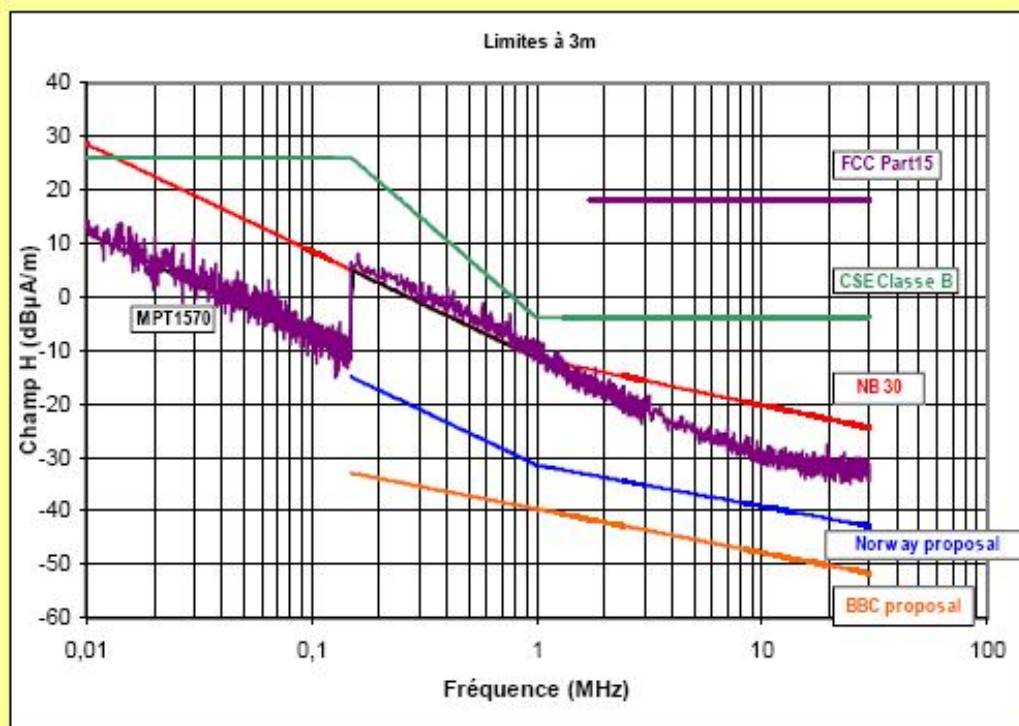
Рис.3.1 Нормовані в різних країнах граничні залежності рівня перешкоди від частоти
