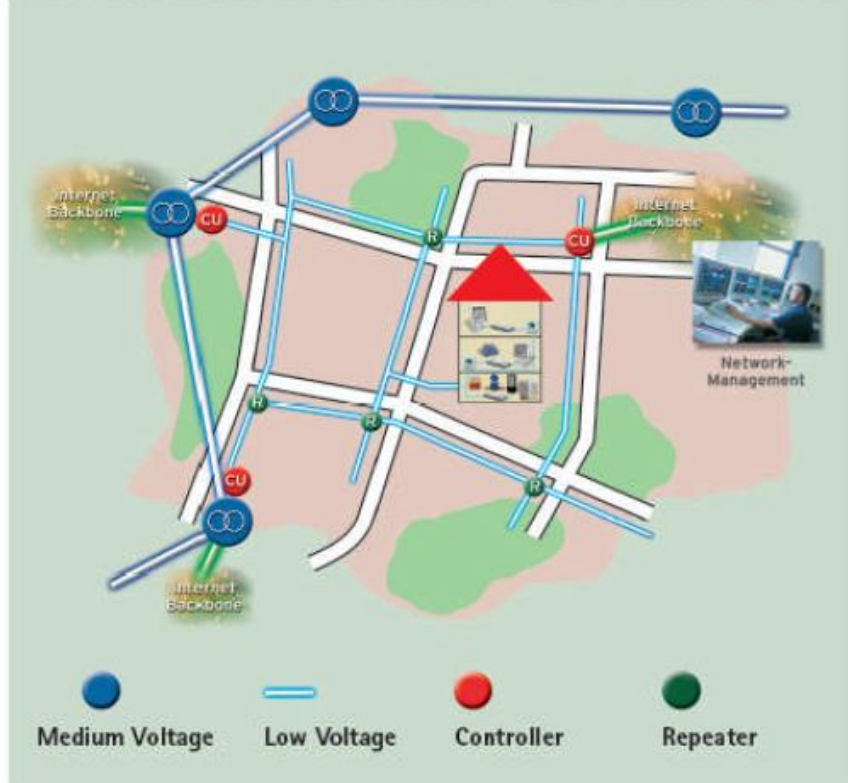
Рис. 1.10 Варіант організації мережі доступу на основі PLC
